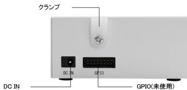
図 1-b 筐体背面
