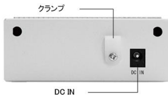
図 1-d 筐体背面
