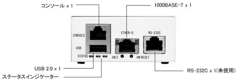
図 1-a 筐体前面
