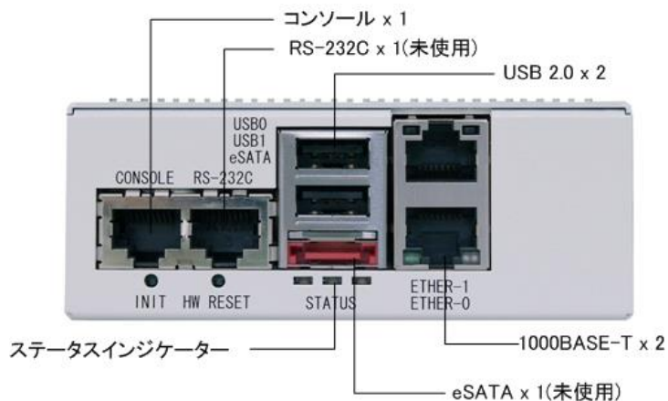
図 1-c 筐体前面
